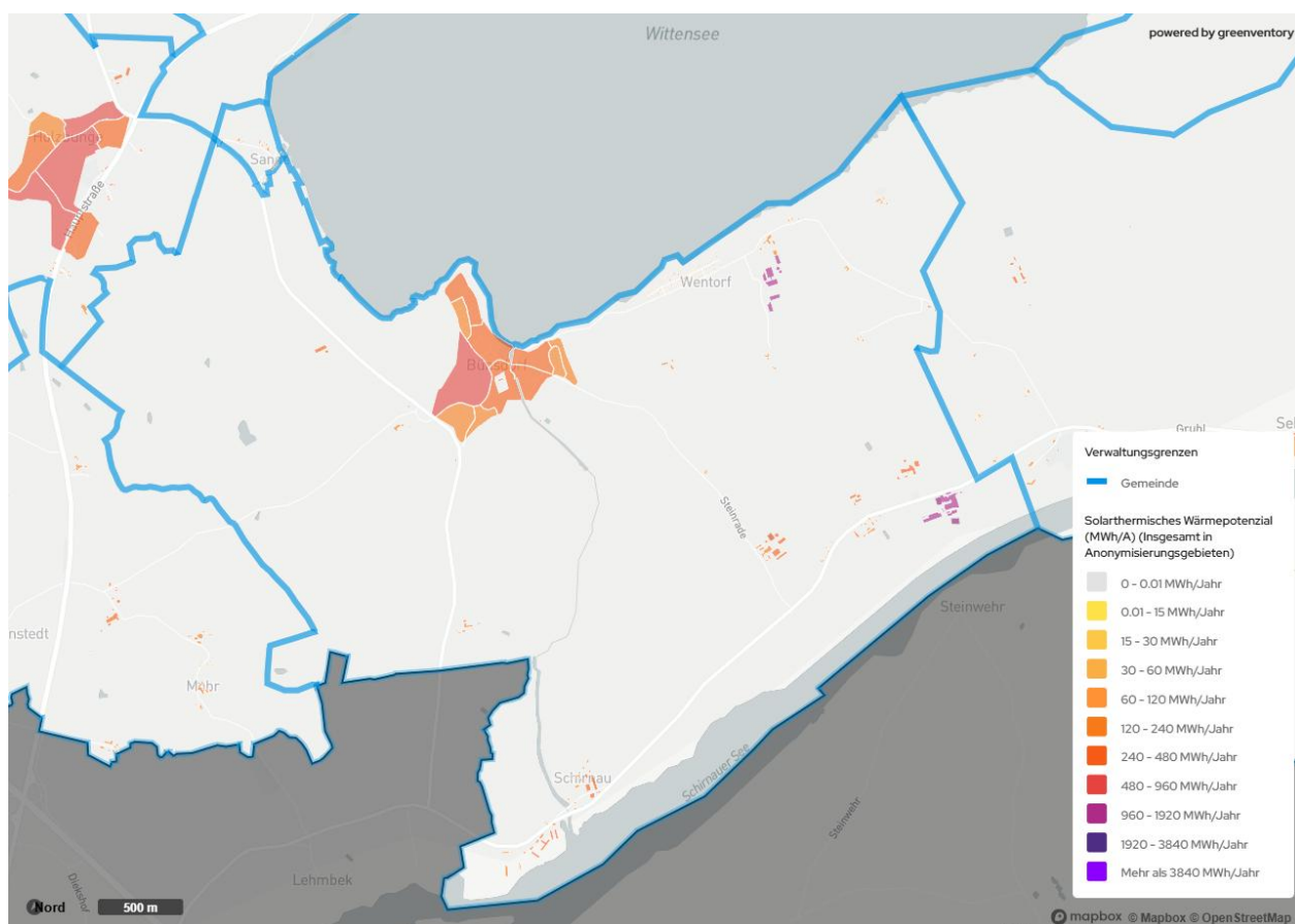
Abbildung 4-10: Potenzial für Solarthermie auf Dachflächen nach Baublock
