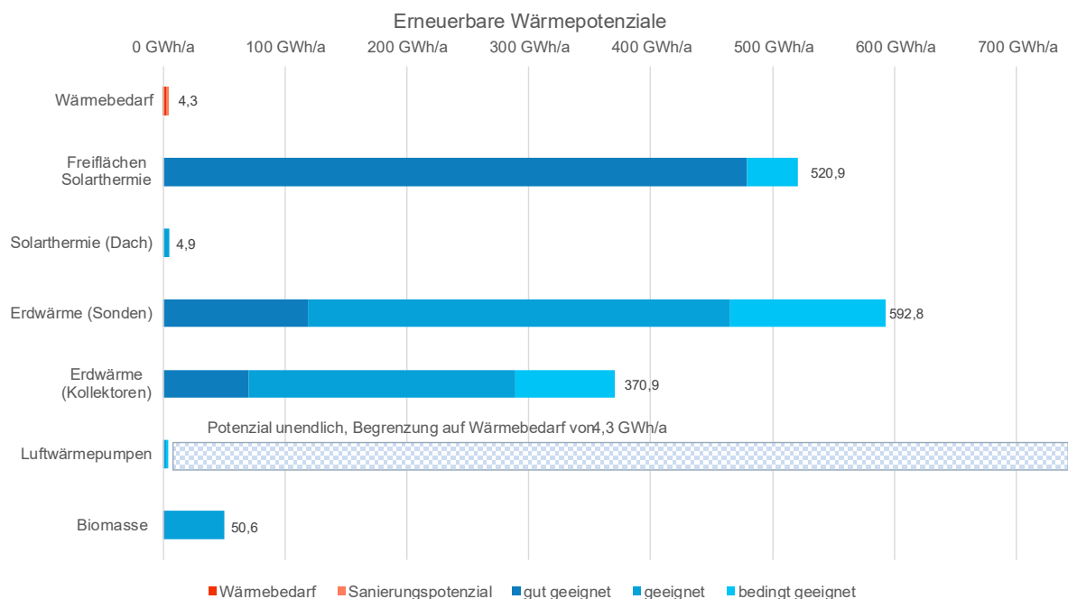
Abbildung 4-8: Erneuerbare Wärmepotenziale im Projektgebiet
