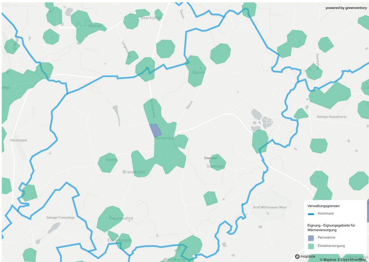
Abbildung 6-3: Versorgungsszenario im Zieljahr 2040 (blau: zentrale Wärmeversorgung, grün: dezentrale Wärmeversorgung)
