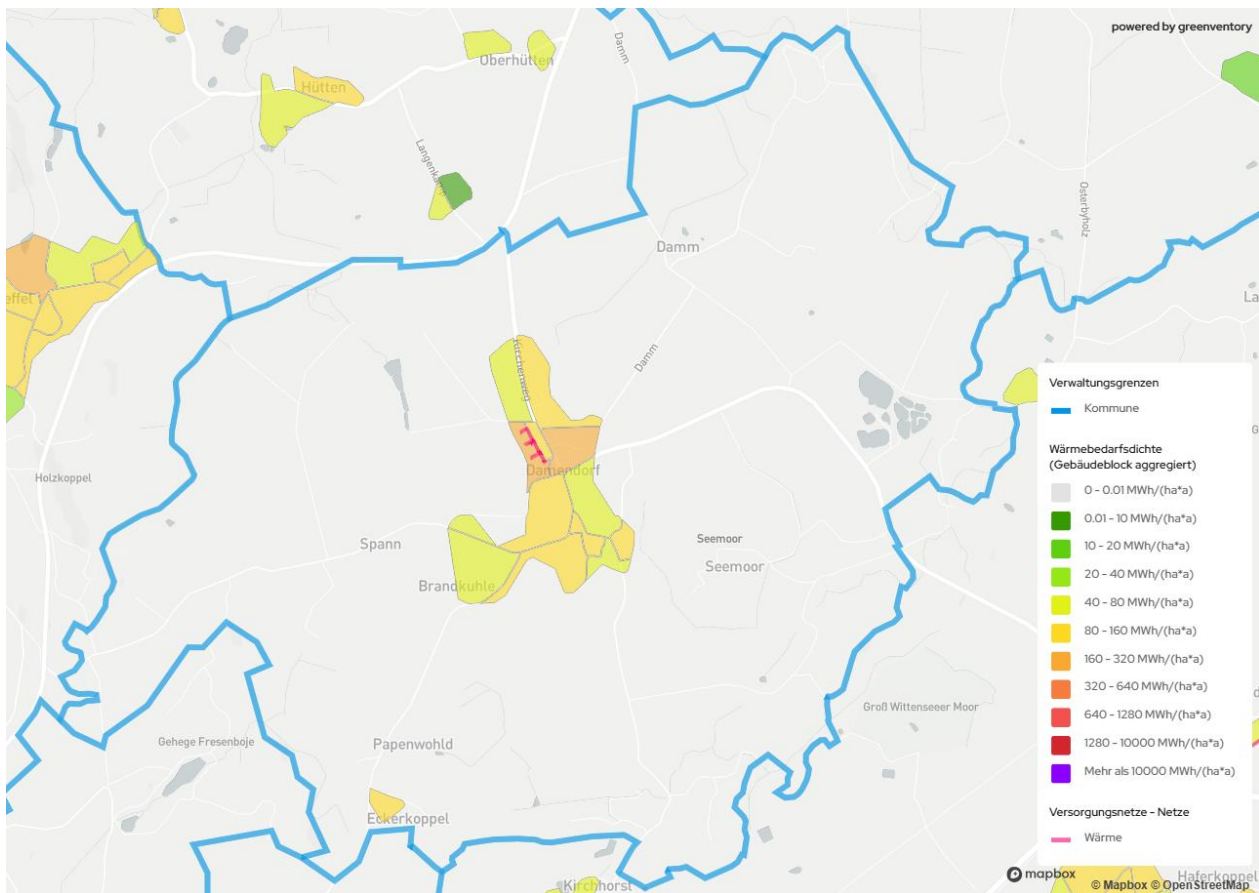
Abbildung 5-4: Wärmebedarfsdichte und bestehendes Wärmenetz
