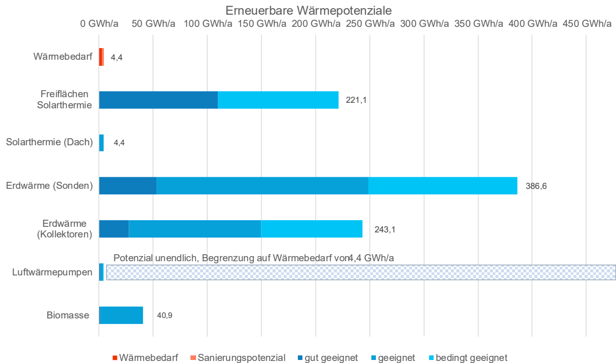
Abbildung 4-8: Erneuerbare Wärmepotenziale im Projektgebiet
