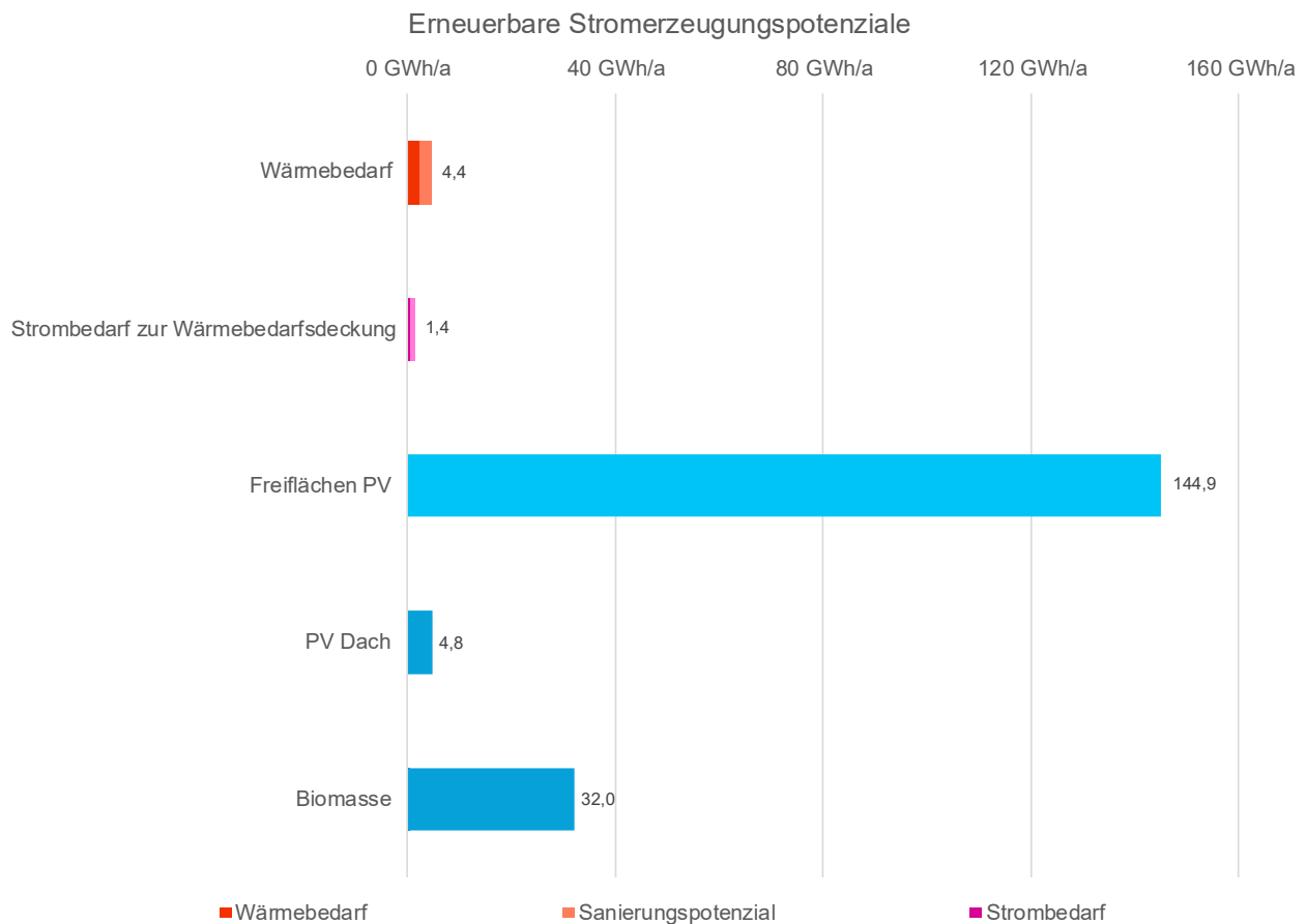
Abbildung 4-4: Erneuerbare Strompotenziale im Projektgebiet
