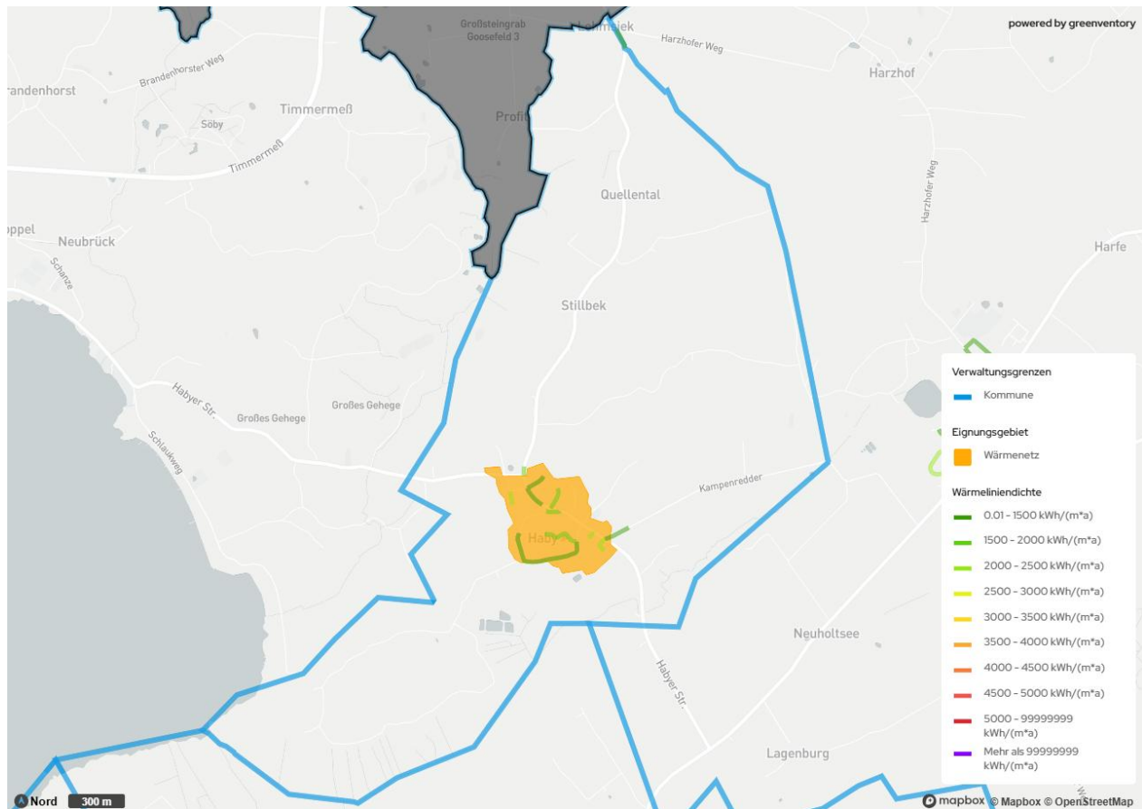
Abbildung 5-6: Prüfgebiete in Ausbaustufe 1 dargestellt über Wärmelinien-dichte ab 1.200 kWh/(m²a)
