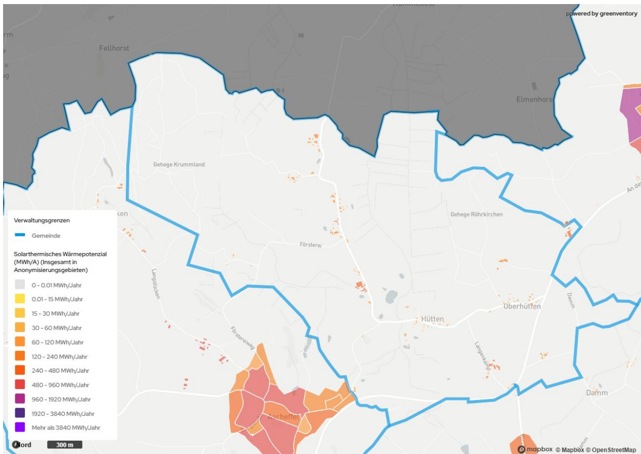
Abbildung 4-10: Potenzial für Solarthermie auf Dachflächen in anonymisierter Form
