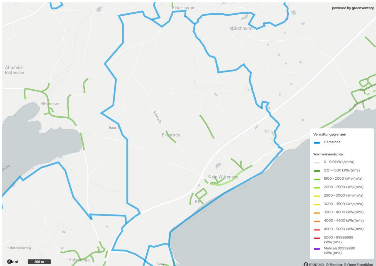
Abbildung 3-16: Wärmelinienindichten
