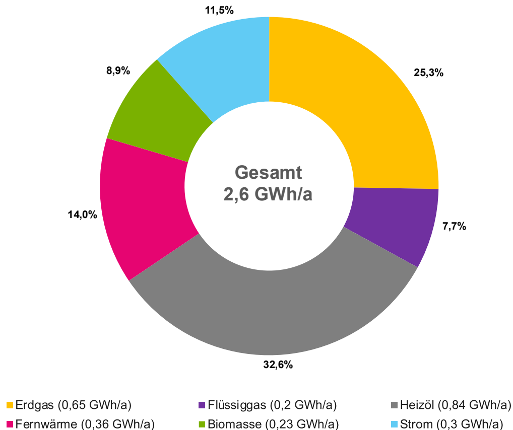
Abbildung 3-13: Energiebedarf nach Energieträger
