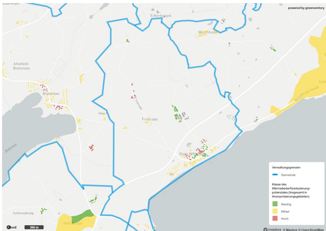
Abbildung 4-16: Sanierungsklassen anonymisiert
