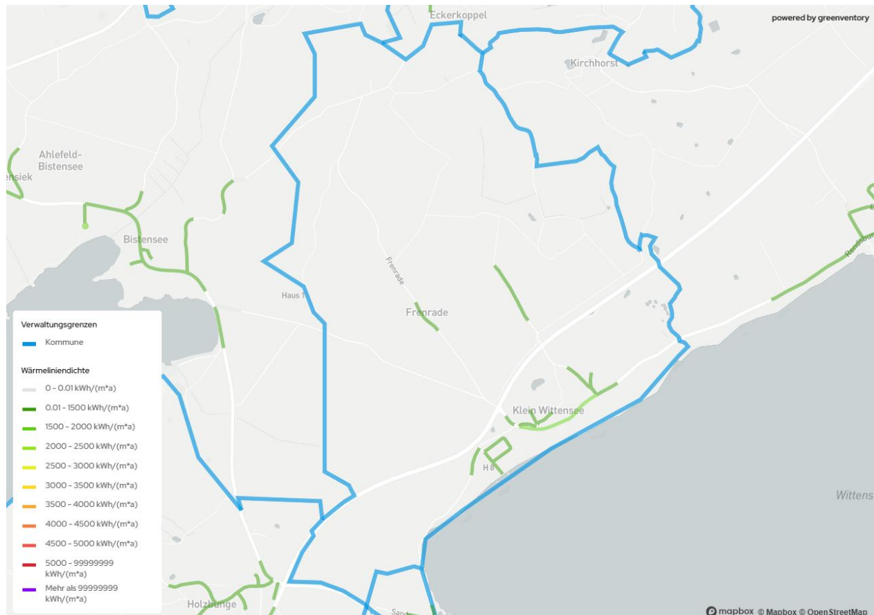
Abbildung 5-3: Wärmeliniedichte
