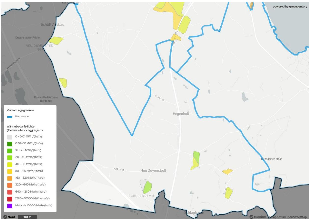
Abbildung 5-4: Wärmebedarfsdichte
