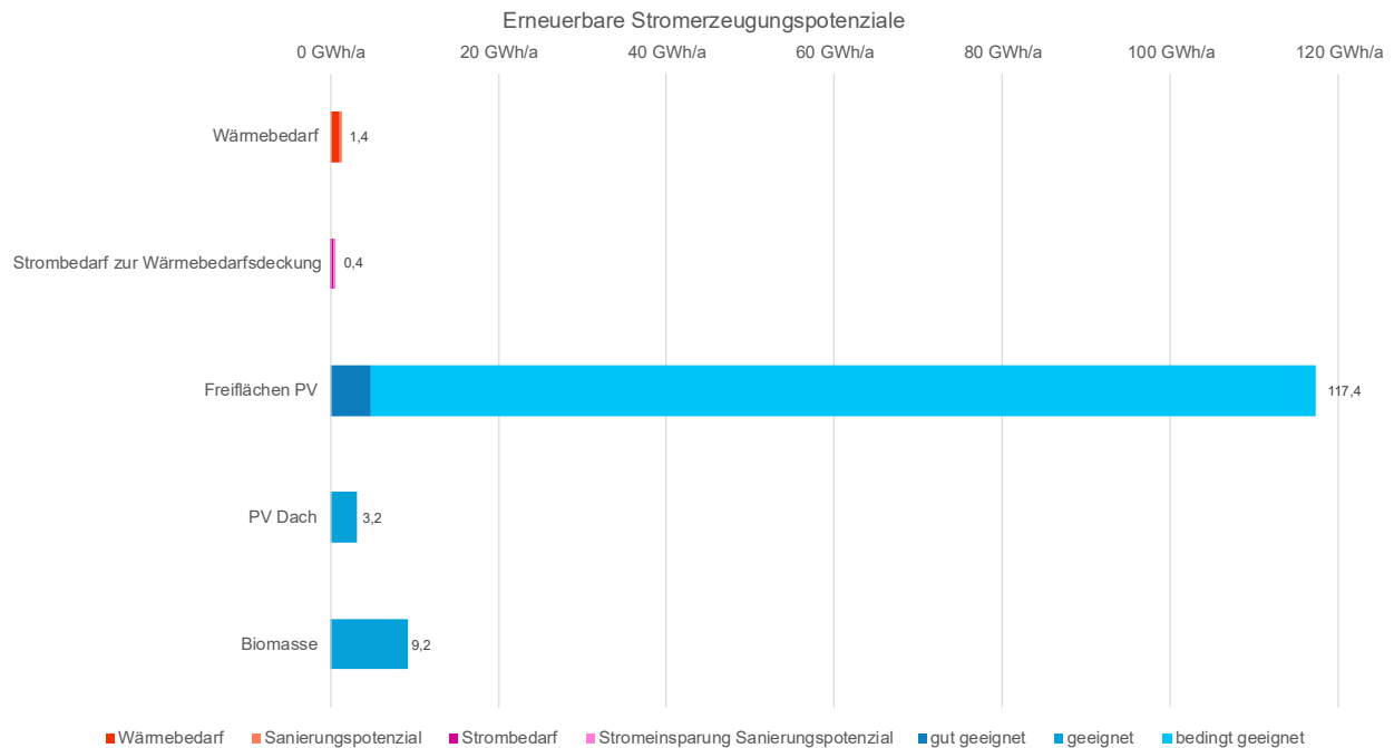
Abbildung 4-4: Erneuerbare Strompotenziale im Projektgebiet
