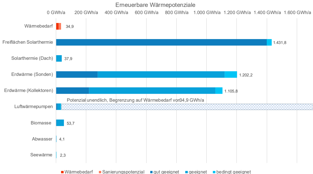
Abbildung 4-9: Erneuerbare Wärmepotenziale im Projektgebiet
