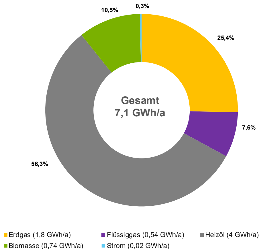
Abbildung 3-13: Energiebedarf nach Energieträger
