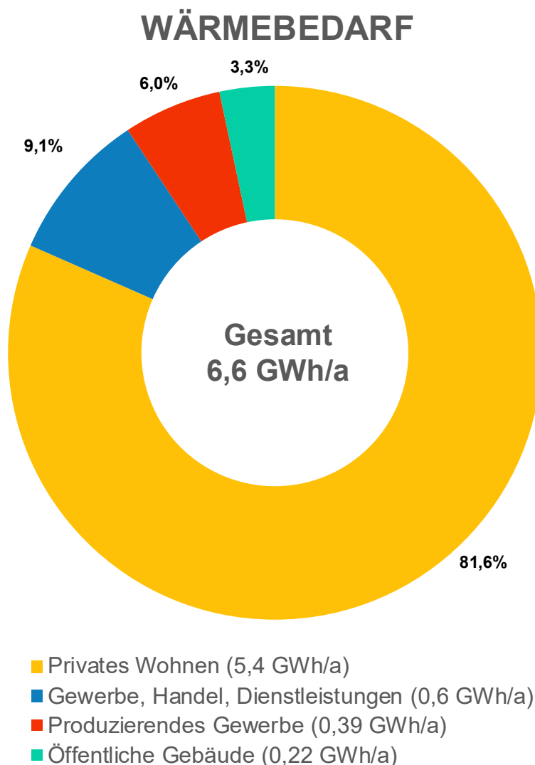
Abbildung 3-8: Wärmebedarf nach Sektor
